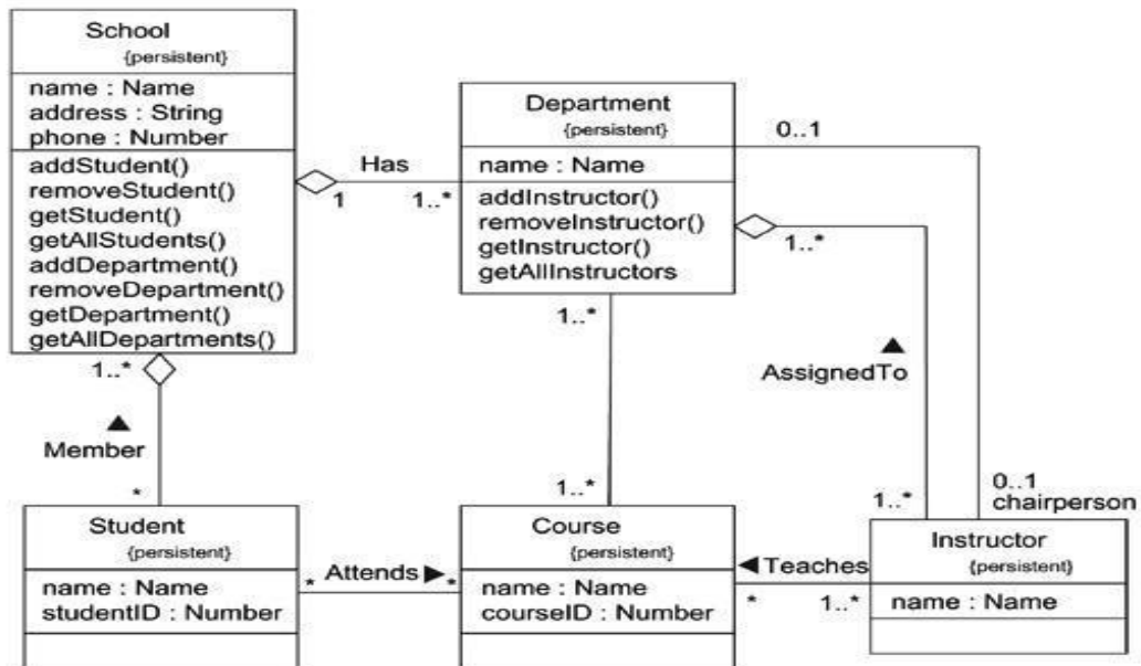
Fig:Modeling a Schema
